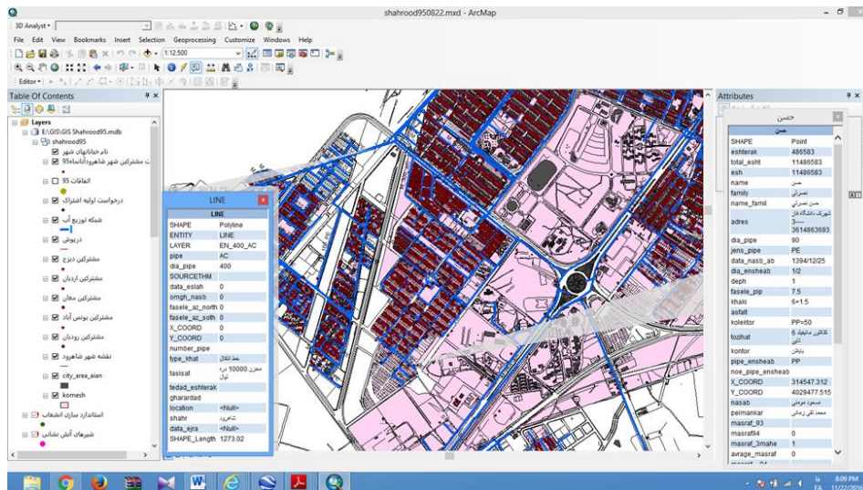
شکل ۲- اطلاعات مشترکین و شبکه توزیع
